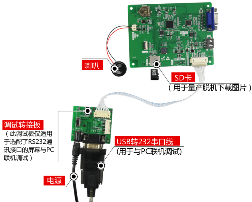
图 1-3 调试工具图
